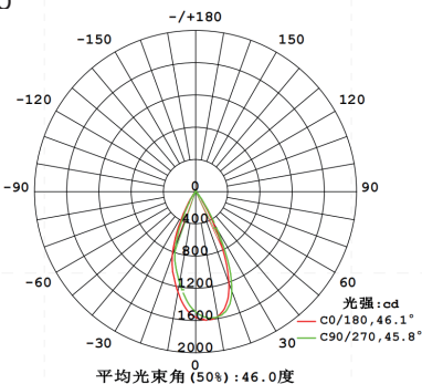
配光曲线图
