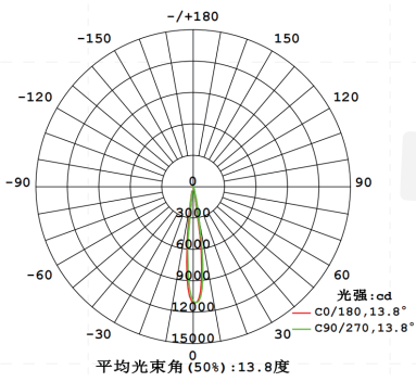
配光曲线图
