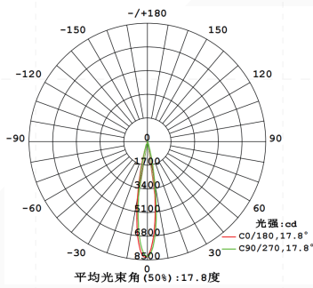
配光曲线图
