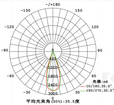
配光曲线图
